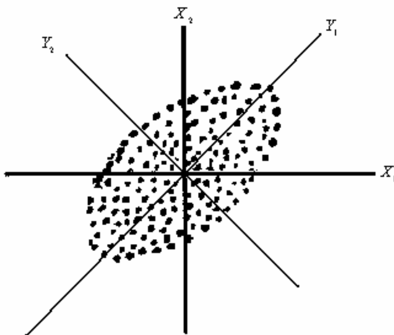
图 17-115 主成分的几何意义
