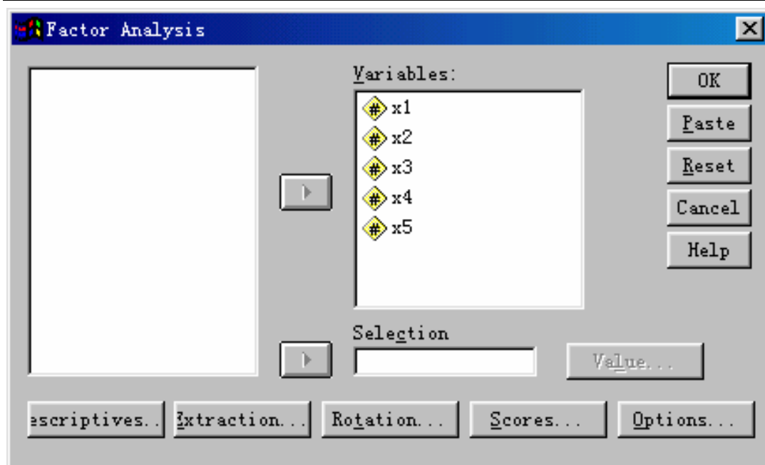
图 18-119 因子分析主对话框
