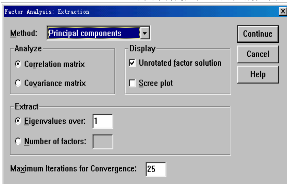
图 13-118 因子提取方法子对话框
