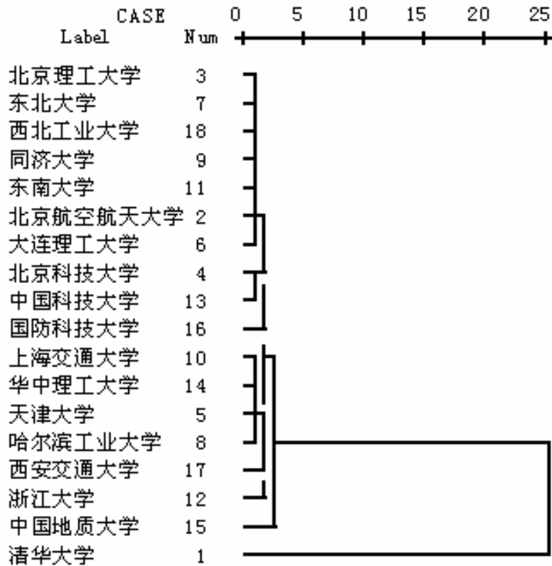
图 18-121 18 所大学研究生院的系统聚类图
