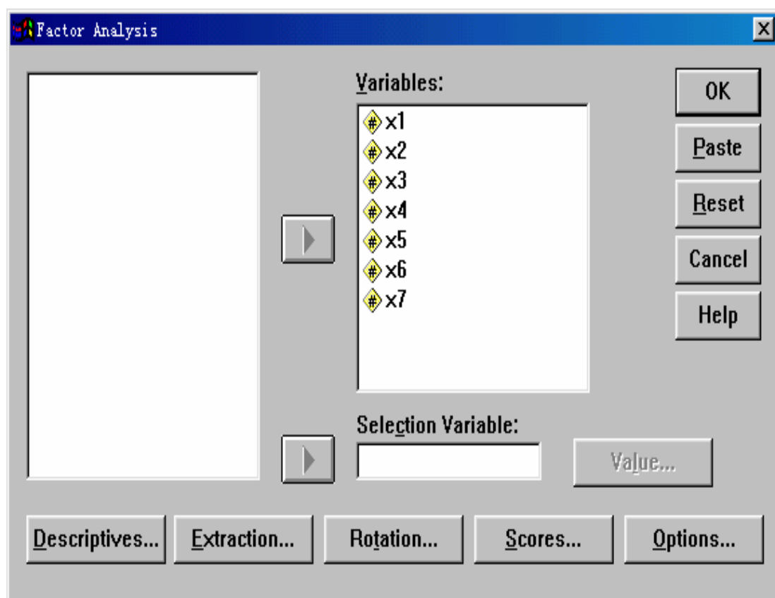
图 13-116 主成分/因子分析主对话框
