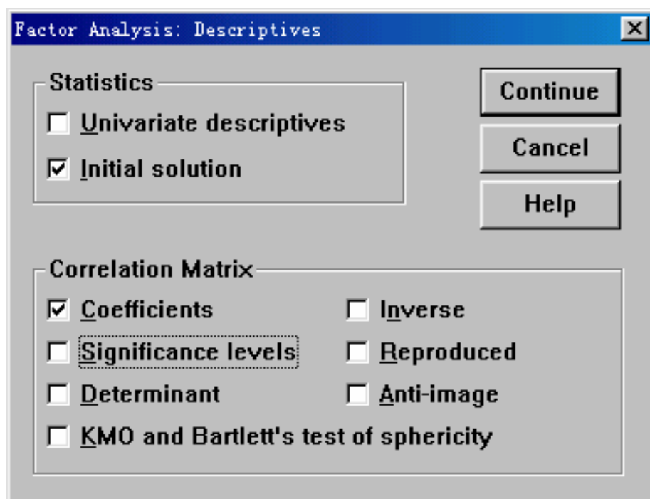
图 13-117 描述统计量子对话框
