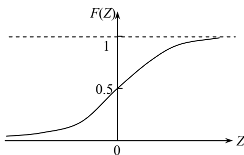
图 4-51 标准正态分布的分布函数图
