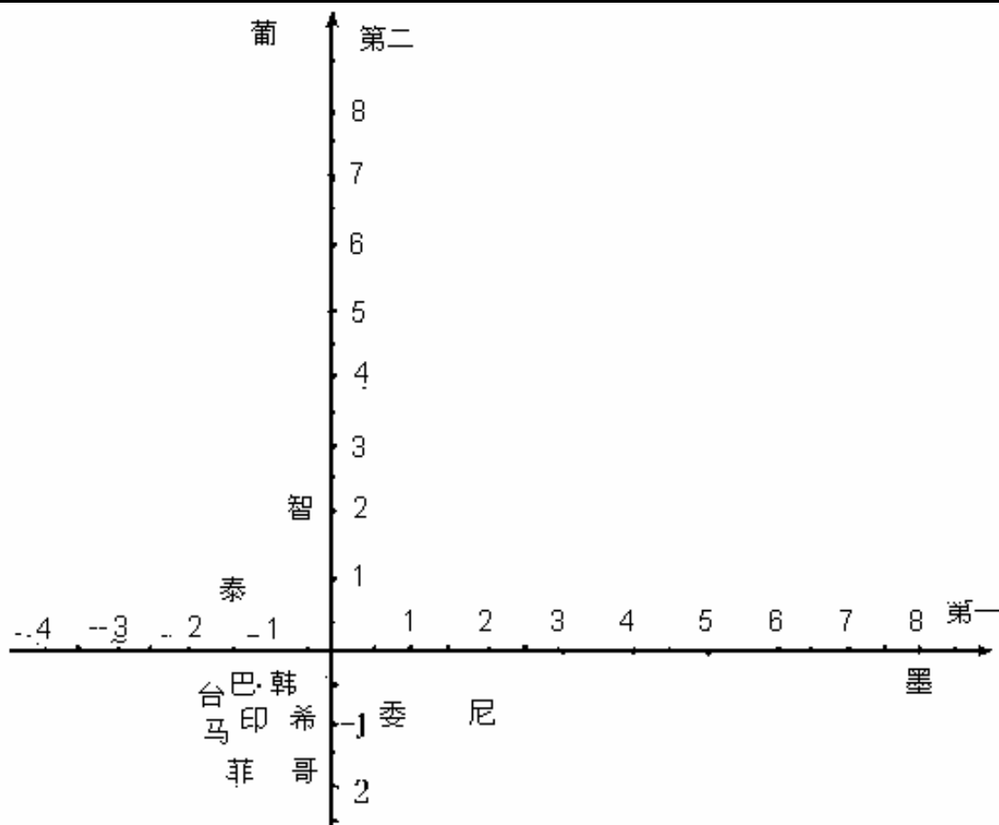
附图 第一、第二主成份点图
